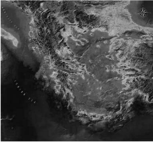
Εικόνα 26.3: Κατανομή των επικέντρων των επιφανειακών σεισμών στον ελληνικό χώρο (Parazachos B.C. et al, 1997)
